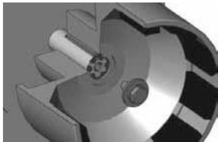
Figura 6 - Motor IEC
